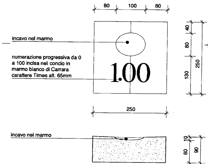
Particolare costruttivo del Concio di supporto per l'alloggiamento e numerazione della famosa "Corsa delle uova"
